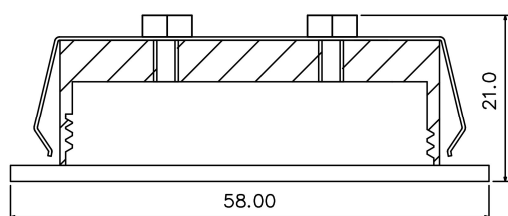
OUTER DIMENSIONS Unit:mm
