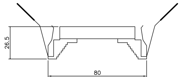
套件外觀尺寸
